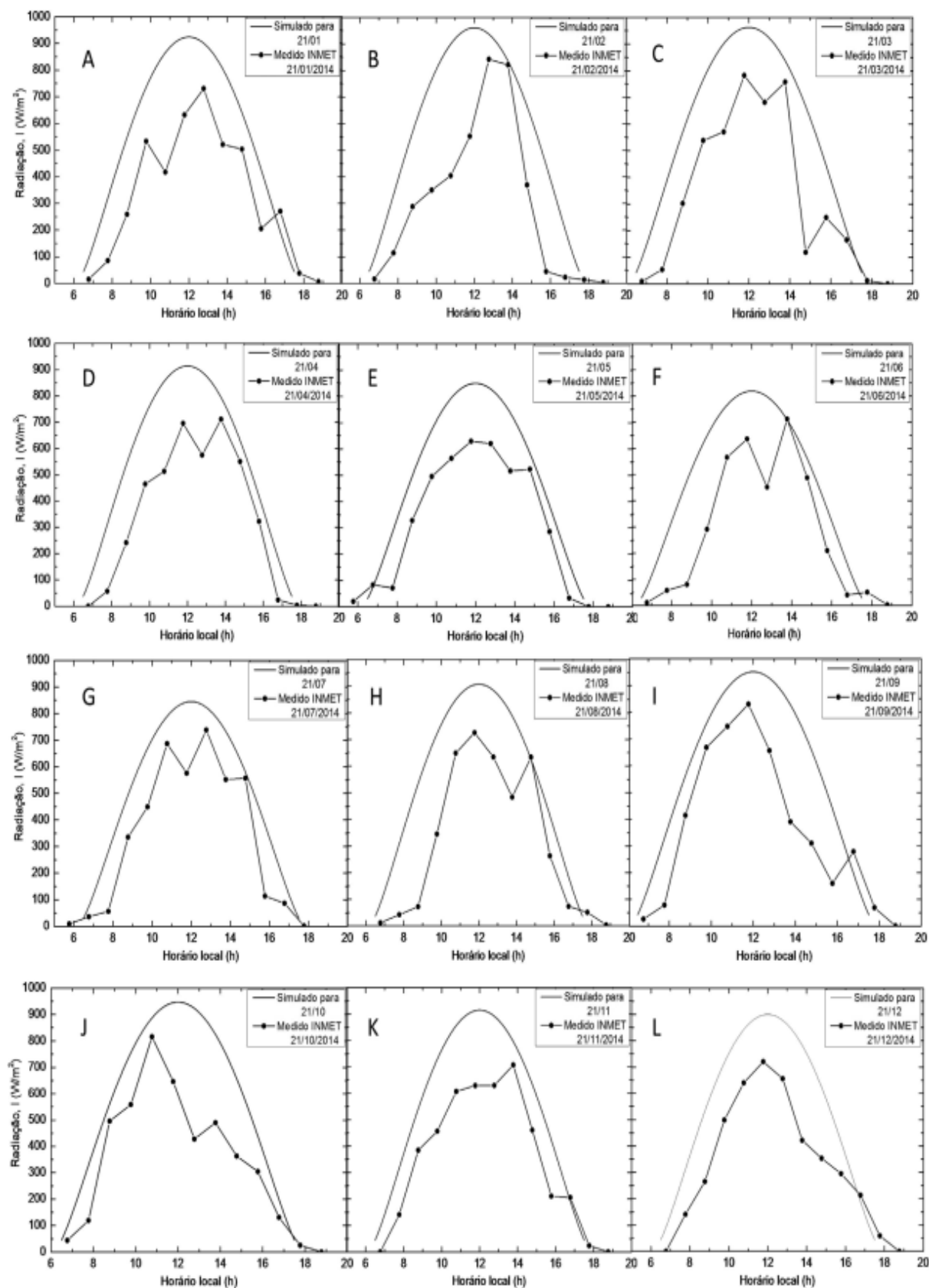
Anexo 1: Radiação simulada no MATLAB vs. Radiação medidas pela estação do INMET- 2014 (CAMPOS; ALCANTARA, 2016).
