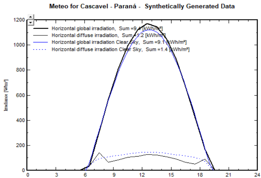
Anexo 11: Gráficos de valores horários para a radiação solar sintéticos (PVSYST, 2020).
