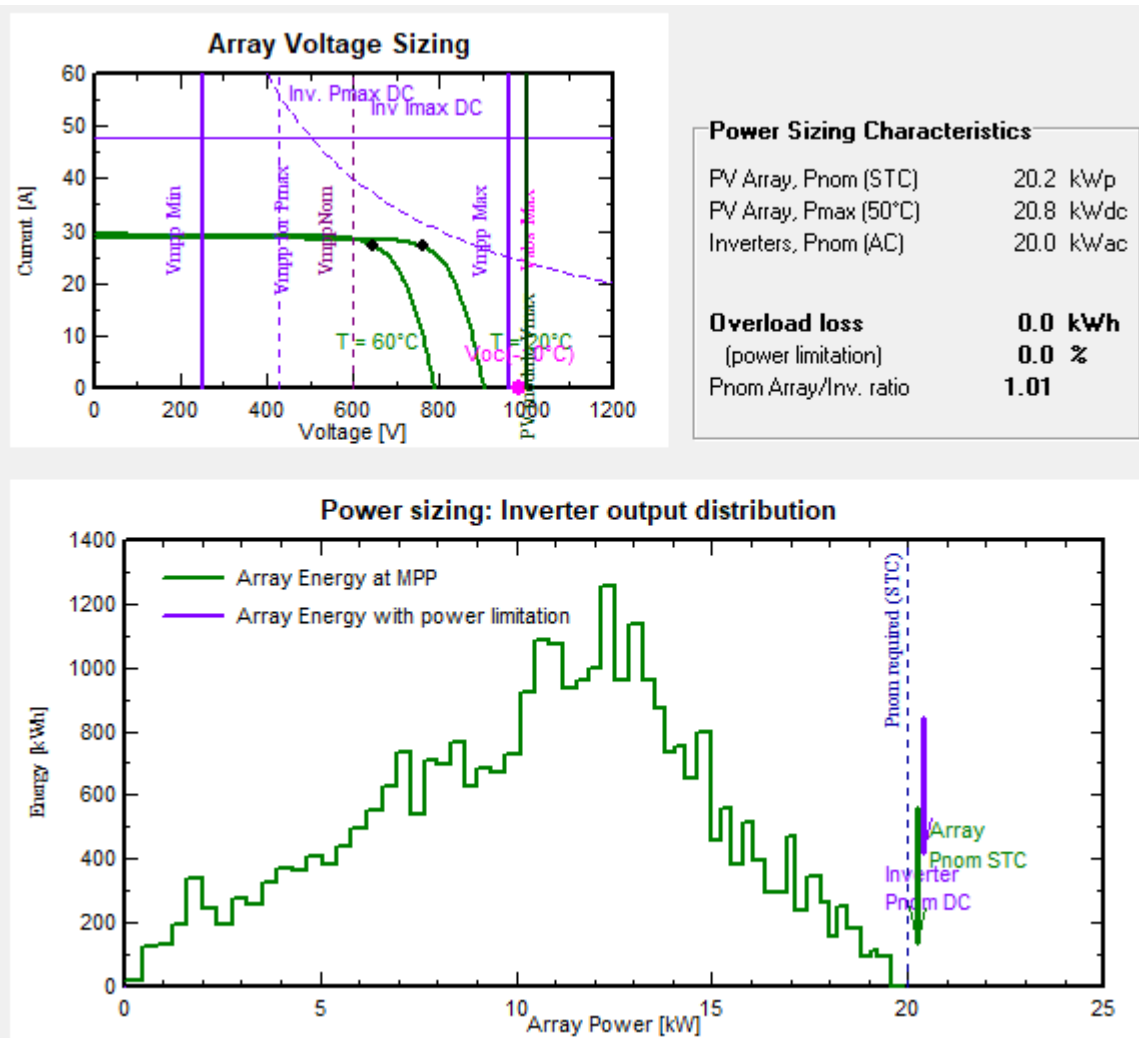
Anexo 17: Dimensionamento do Inversor para o sistema de 20kWp (PVSYST, 2020).
