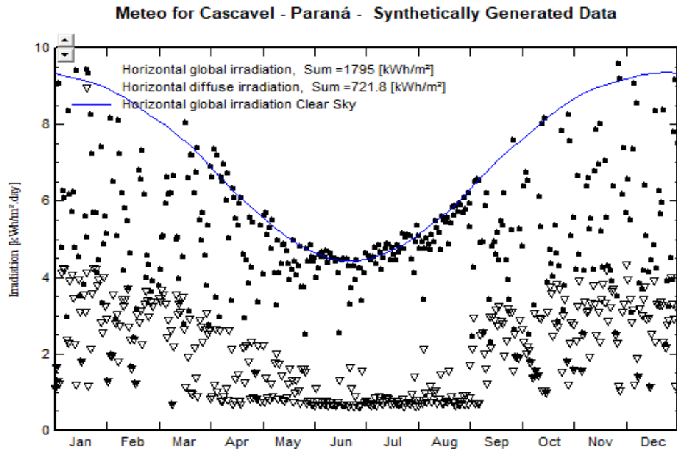
Anexo 10: Dados de distribuição anual sintéticos (PVSYST, 2020).
