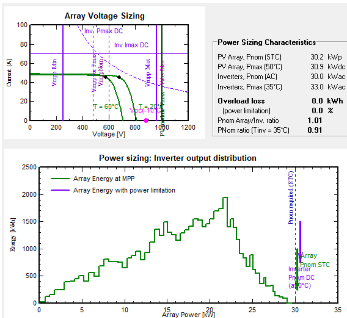
Anexo 19: Dimensionamento do Inversor para o sistema de 30kWp (PVSYST, 2020).
