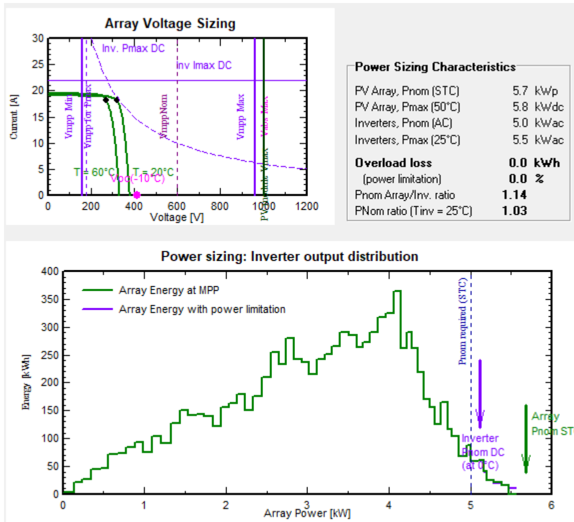
Anexo 13: Dimensionamento do Inversor para o sistema de 5kWp (PVSYST, 2020).
