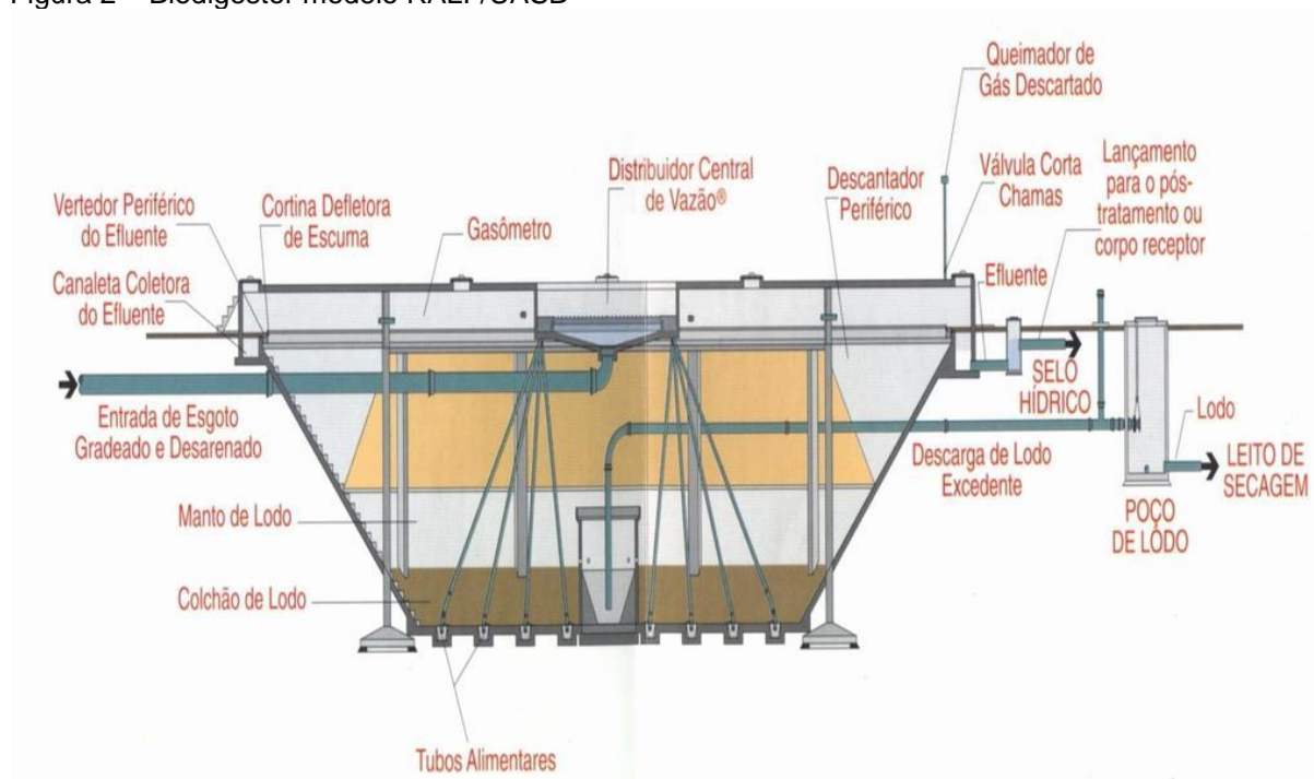
Figura 2 – Biodigestor modelo RALF/UASB
