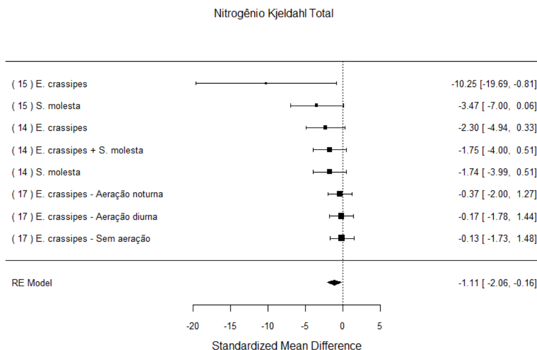
Fig. 9 Metanálise do nitrogênio Kjeldahl total elaborado a partir das médias e desvios padrões nos tratamentos de afluentes com macrófitas flutuantes. Onde, aeração diurna, aeração noturna e sem aeração equivalem ao tipo de tratamento. Os números entre parênteses se referem a coluna de ordem cronológica na Tabela 1.
