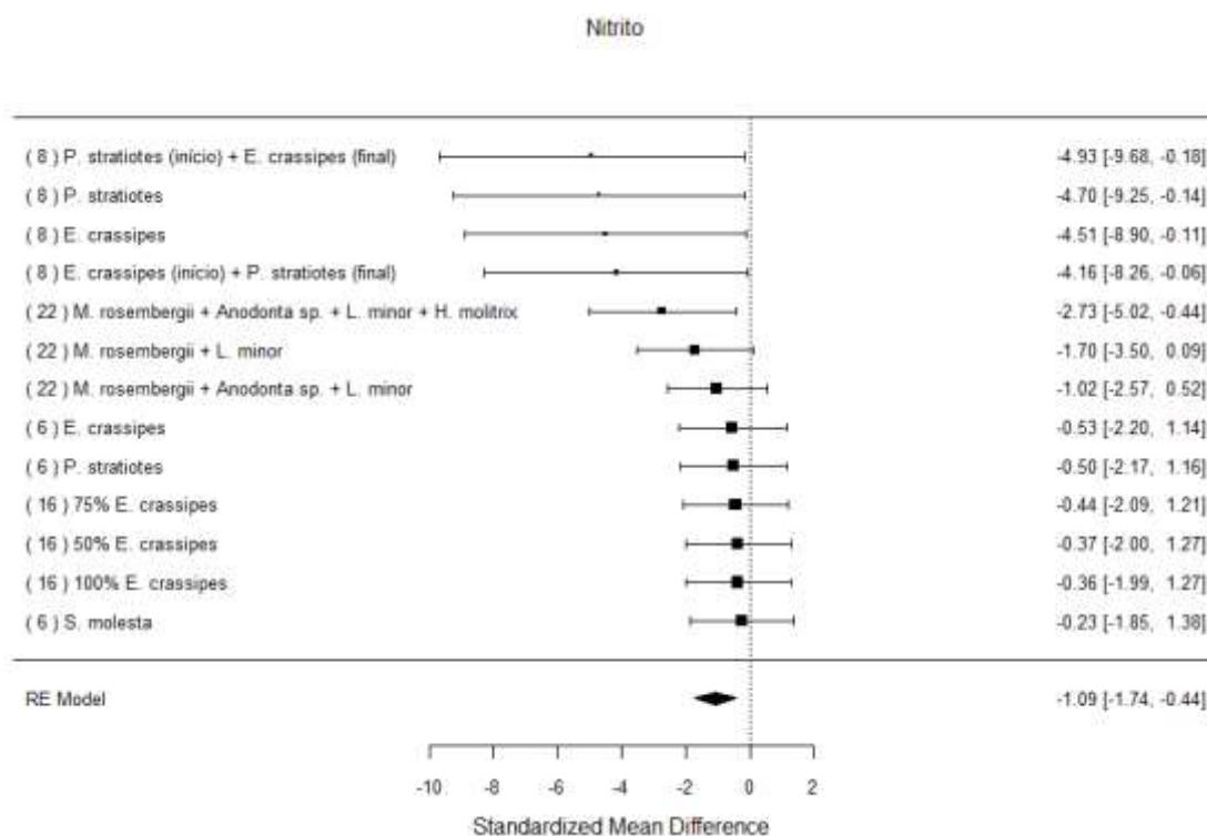
Fig. 7 Metanálise do nitrito a partir das médias e desvios padrões nos tratamentos de efluentes com macrófitas flutuantes. Onde, 50%, 75% e 100% representam a porcentagem de cobertura vegetal na superfície do tanque experimental. Início e final são as posições ocupadas pelas macrófitas no viveiro. Os números entre parênteses se referem a coluna de ordem cronológica na Tabela 1.
