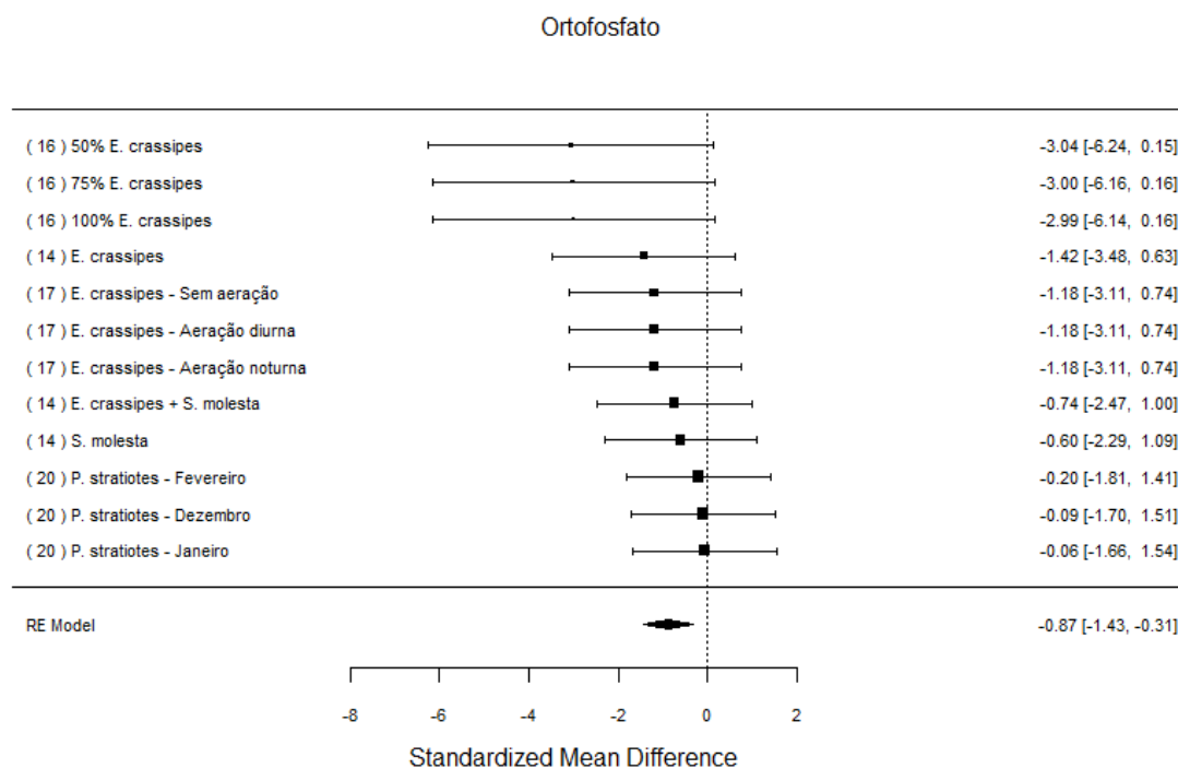
Fig. 12 Metanálise do ortofosfato elaborado a partir das médias e desvios padrões nos tratamentos de efluentes com macrófitas flutuantes. Onde 50%, 75% e 100% representam a porcentagem de cobertura vegetal na superfície do tanque experimental. Aerção diurna, aerção noturna e sem aerção equivalem ao tipo de tratamento. Os números entre parênteses se referem a coluna de ordem cronológica na Tabela 1.
