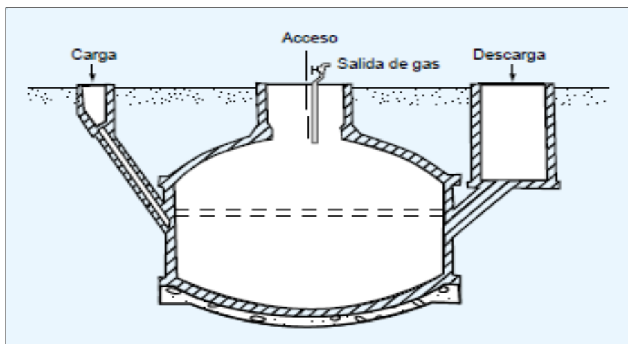
Figura 7 - Modelo de Biodigestor – Chinês
