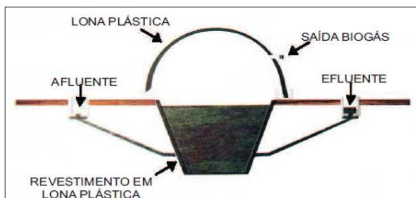
Figura 8 - Modelo de biodigestor – Canadense
