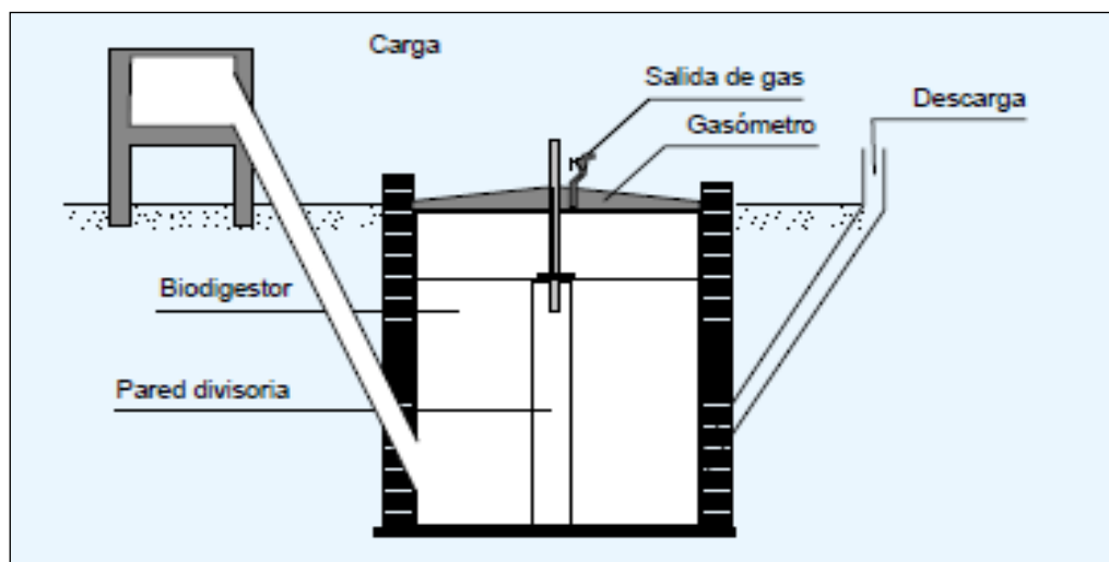
Figura 6 - Modelo de Biodigestor – Indiano
