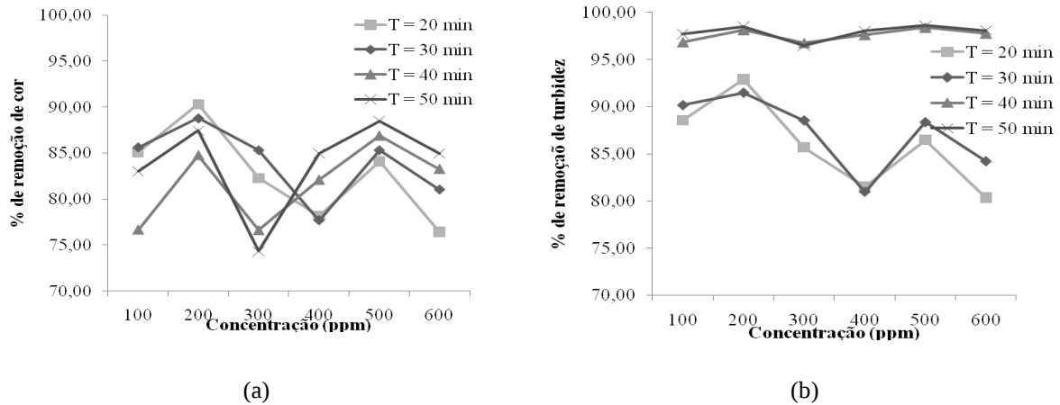
Figura 6. Porcentagem de remoção de cor (a) e turbidez (b) em tempos de sedimentação distintos utilizando sementes de moringa em diferentes concentrações
