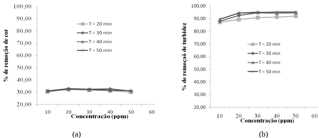
Figura 4. Porcentagem de remoção de cor (a) e turbidez (b) em tempos de sedimentação distintos utilizando cloreto férrico em diferentes concentrações
