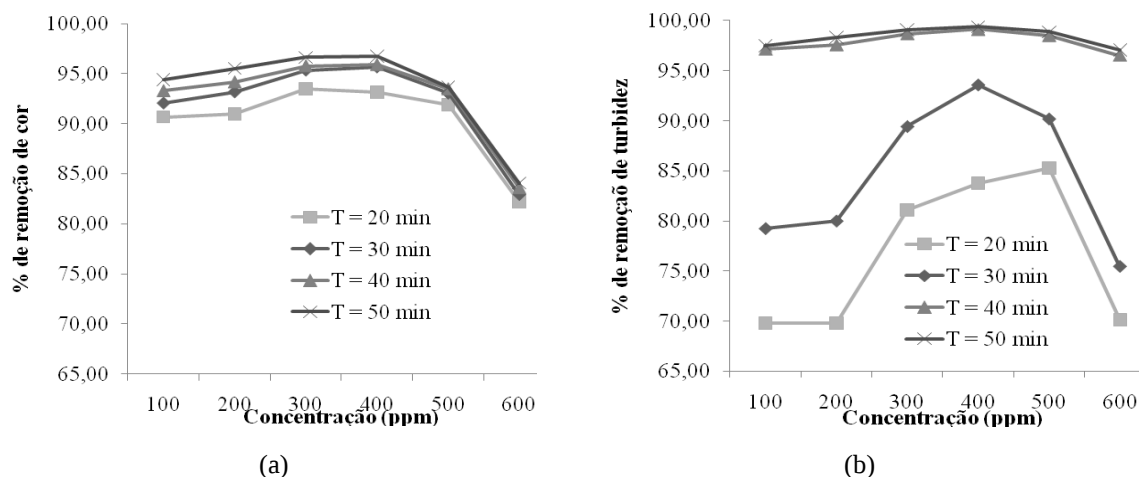
Figura 7. Porcentagem de remoção de cor (a) e turbidez (b) em tempos de sedimentação distintos utilizando Tanfloc SG em diferentes concentrações
