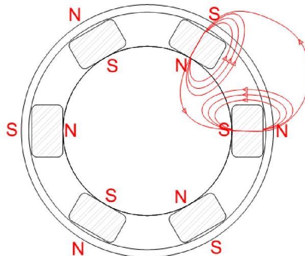
Figura 14 – Planta baixa do rotor magnético composto de seis ímãs com inversão de polos.
