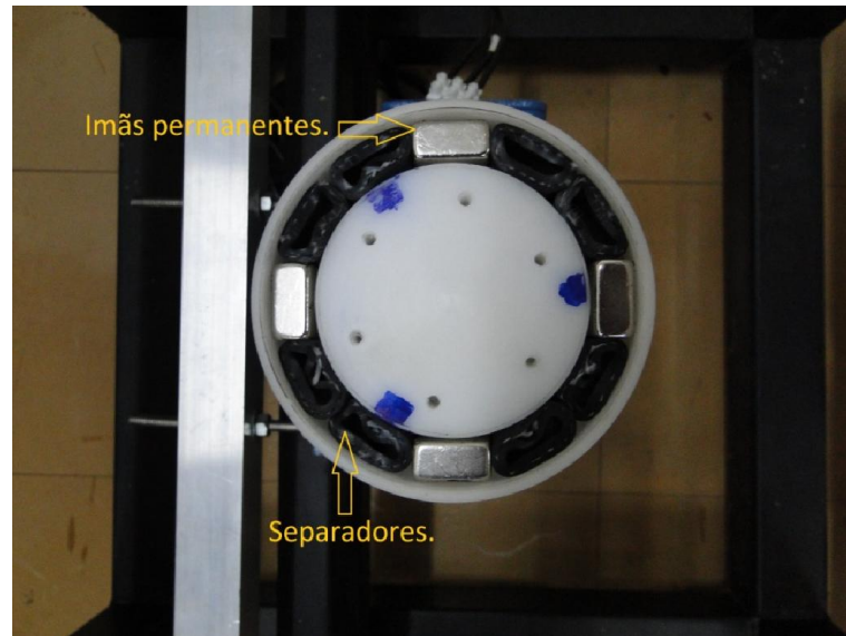
Figura 19 – Detalhe do rotor com quatro ímãs.
