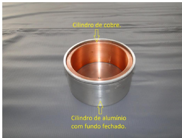
Figura 5 - Gerador/trocador de calor.
