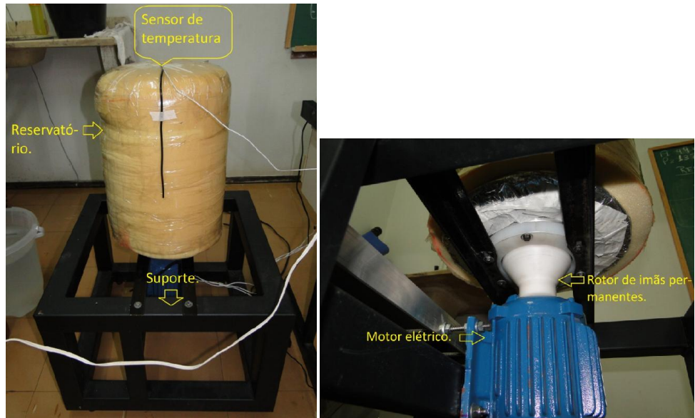
Figura 12 – Vista geral do protótipo.
