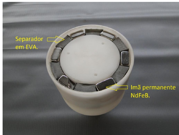
Figura 16 – Detalhe do rotor com seis ímãs.
