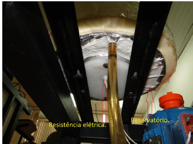
Figura 20 – Detalhe do sistema de aquecimento resistivo.
