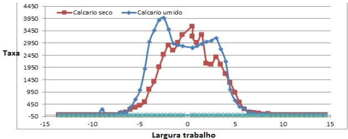
Figura 9. Gráfico comparativo de perfil testes 7 e 8, taxa (kg ha -1 ) em função da largura de trabalho (m.).
