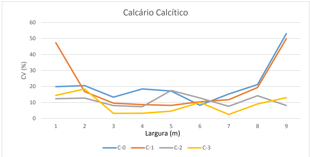
Figura 16. Gráfico de CV% do perfil longitudinal, para o calcário calcítico nas diferentes umidades: C-0 menor teor de umidade; C-1 teor intermediário 1; C-2 teor intermediário 2; C-3 maior teor umidade.
