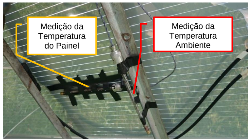
Figura 18. Termopares instalados na face inferior e na sombra do painel.
