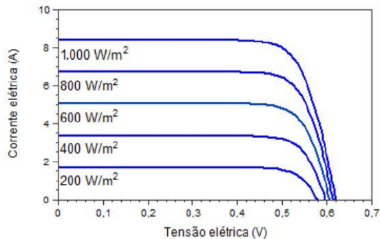
Figura 6. Curva I-U de uma célula fotovoltaica de silício cristalino à 25°C. Fonte: CRESESB (2014)
