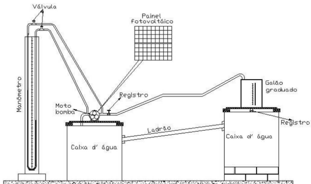
Figura 12 - Diagrama esquemático do sistema com diferentes alturas manométricas. Fonte: Kolling et al. (2004)
