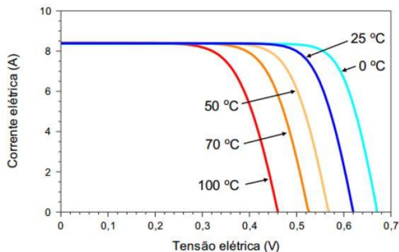
Figura 7. Curvas I-U de uma célula fotovoltaica em diferentes temperaturas à 1000 W m⁻². Fonte: CRESESB (2014)
